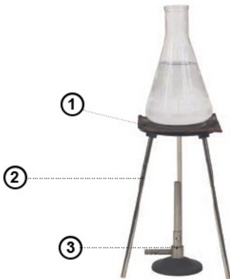
1. wire gauze - la malla metálica 2. tripod - el trípode 3. Bunsen burner - el mechero Bunsen
